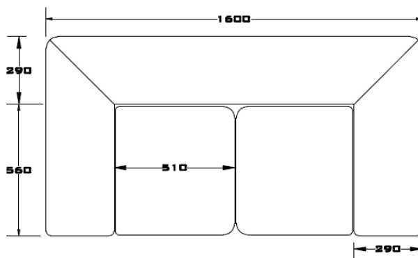
VISTA SUPERIOR
