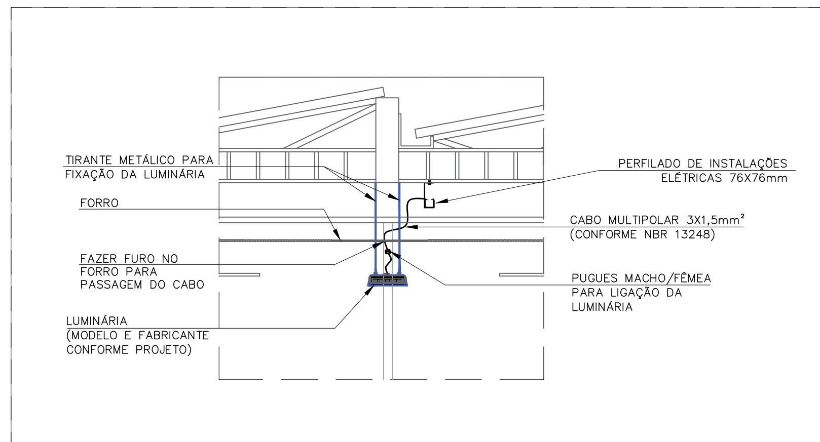
DETALHE - INSTALAÇÃO DE LUMINÁRIA NO TETO DA GALERIA S/ ESCALA
