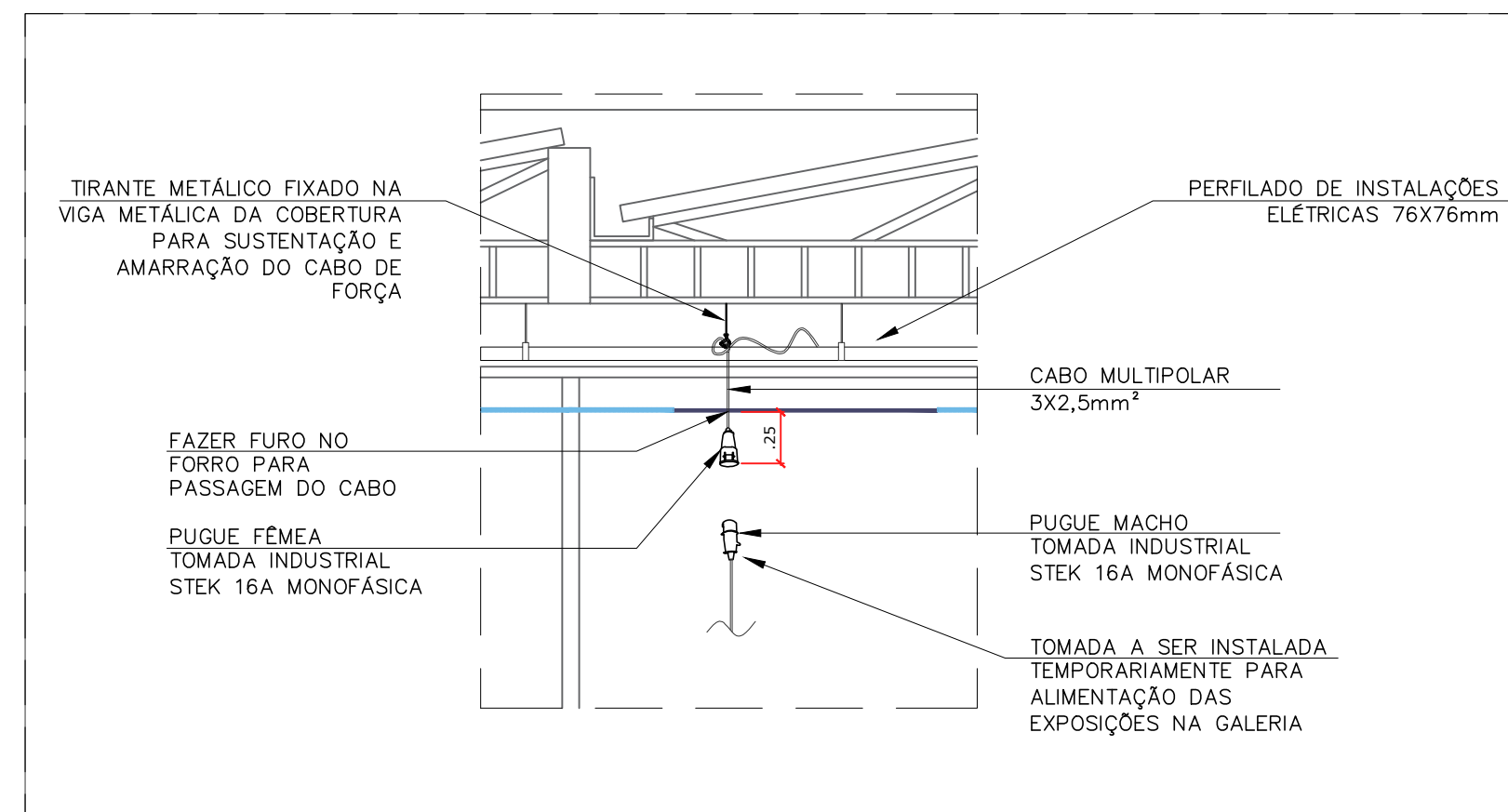
DETALHE - INSTALAÇÃO DE TOMADA INDUSTRIAL NO TETO DA GALERIA S/ ESCALA
