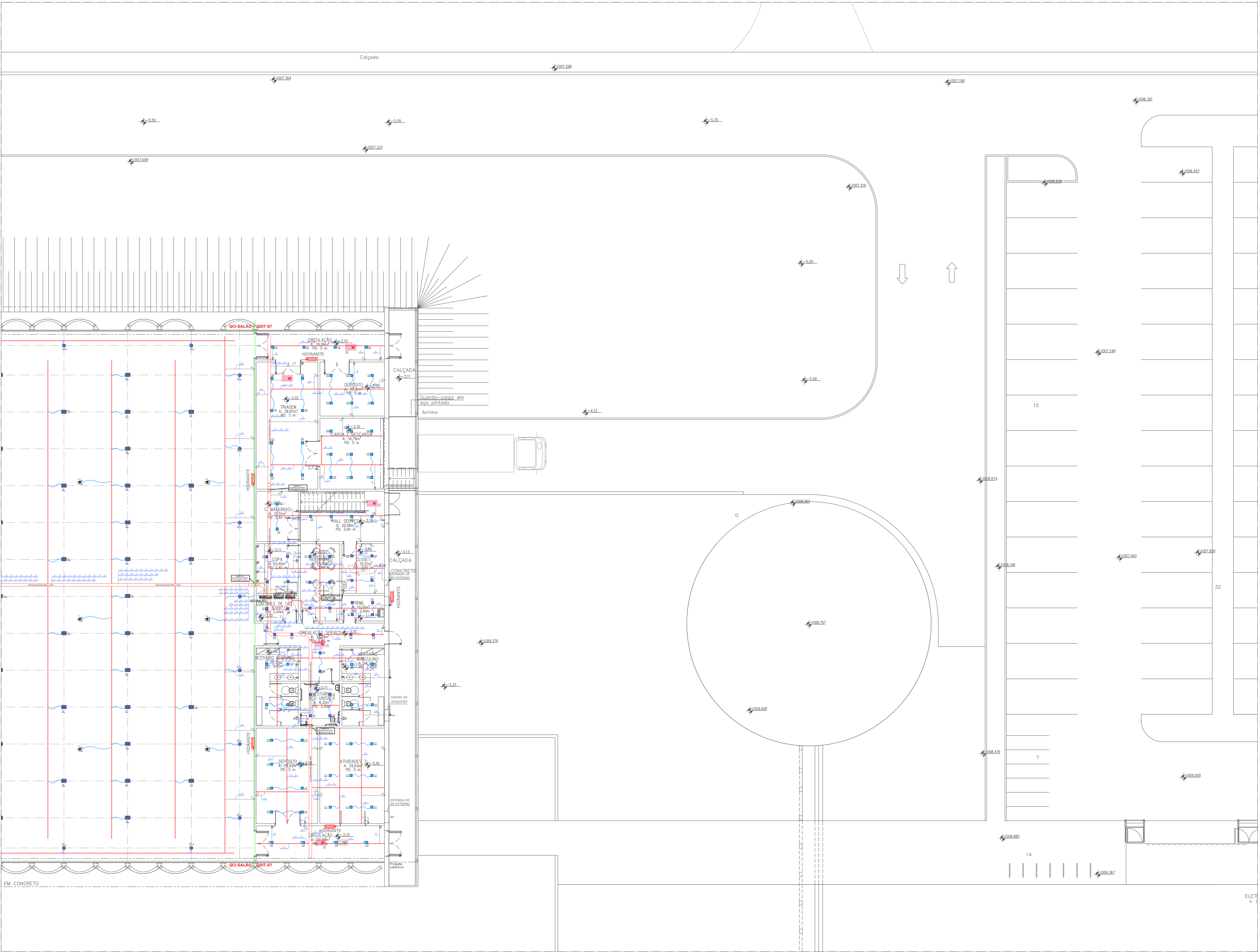
PLANTA BAIXA - SEMIENTERRADO - PARTE 3 ESCALA 1:100
