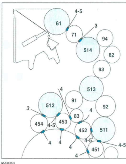
Figura 1 - Esquema de rolos da impressora offset Manroland R708 3B P 4/4
