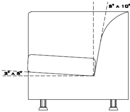
CORTE TRANSVERSAL
