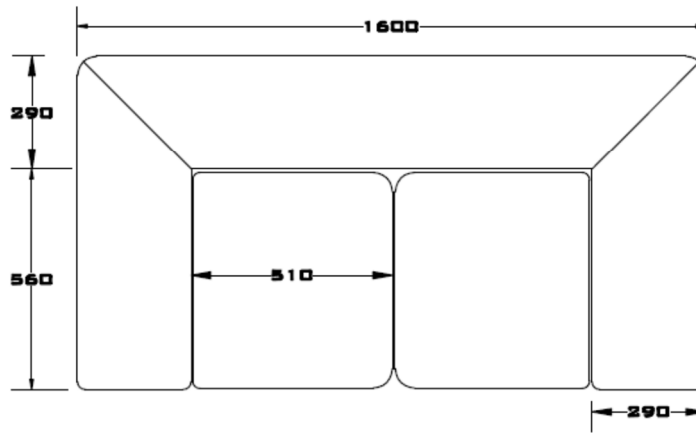
VISTA SUPERIOR
