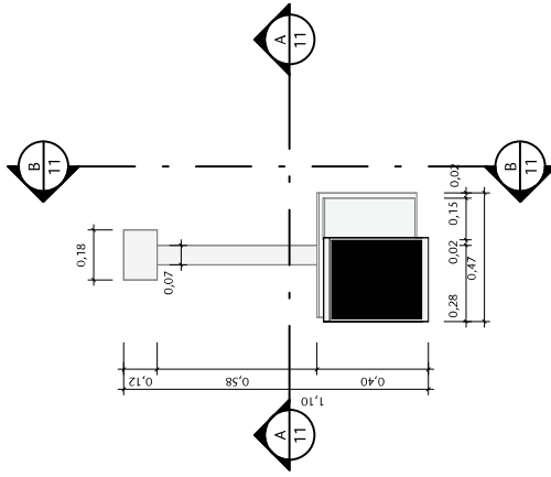
1 DM002 - VISTA SUPERIOR ESCALA 1:20
