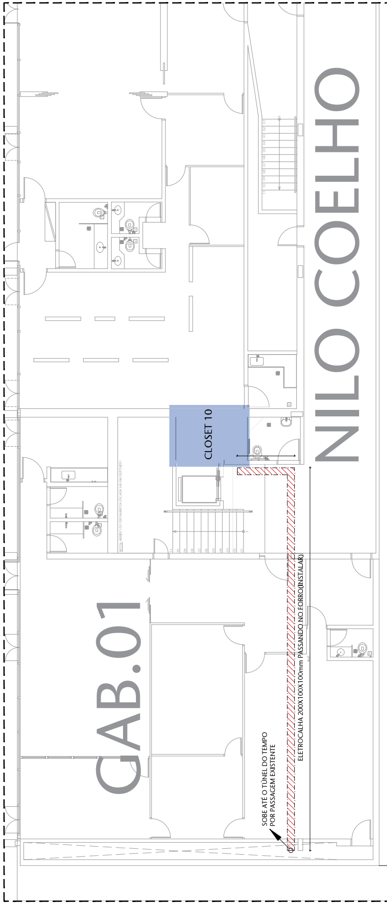
01 PLANTA BAIXA - TÉRREO ALA NILO COELHO ESCALA 1/25
