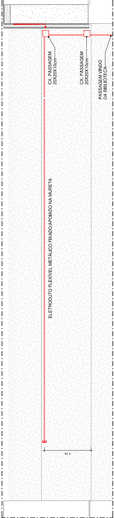
2 Corte 02 ESCALA 1:50
