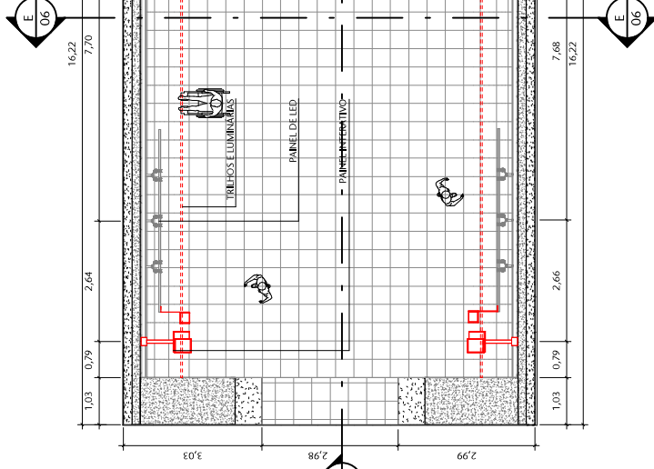
2 SITUAÇÃO PROPOSTA - TRECHO C ESCALA 1 : 100
