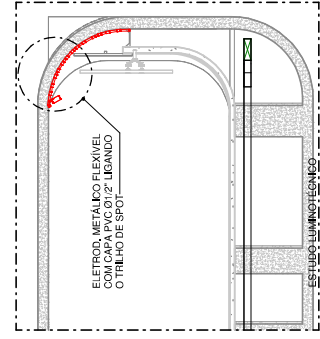
4 - CORTE BBB ESCALA 1:50
