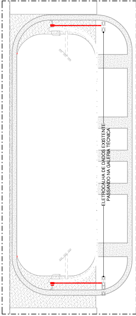
1 Corte 03 ESCALA 1:50
