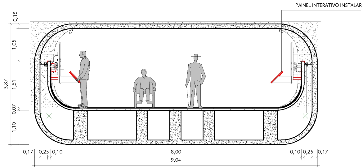
1 CORTE C ESCALA 1 : 75
