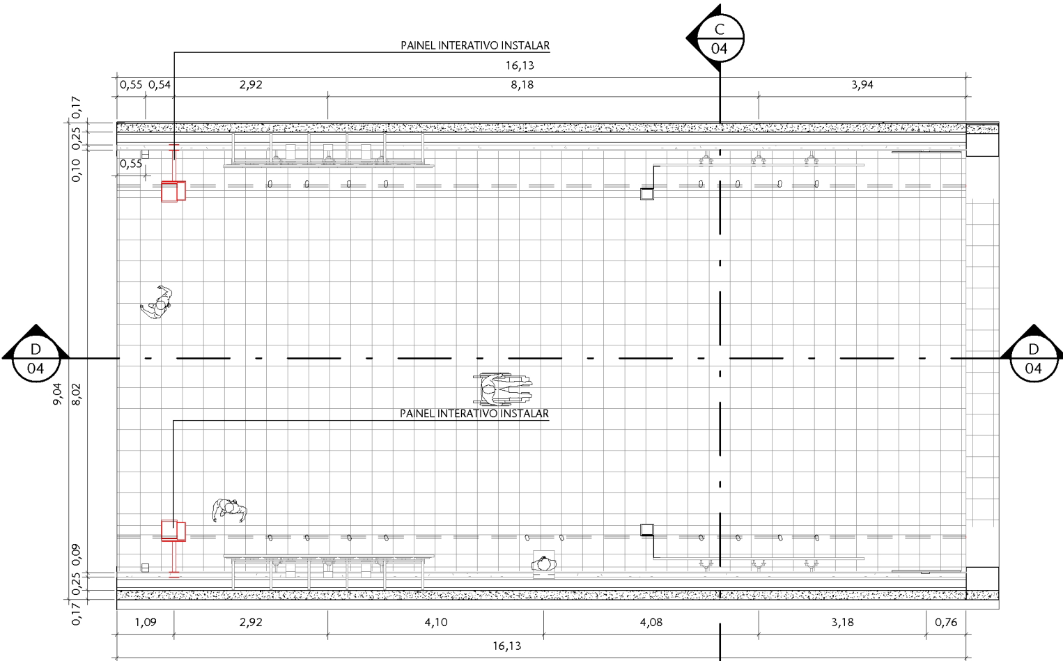
2 SITUAÇÃO PROPOSTA - TRECHO B ESCALA 1 : 100
