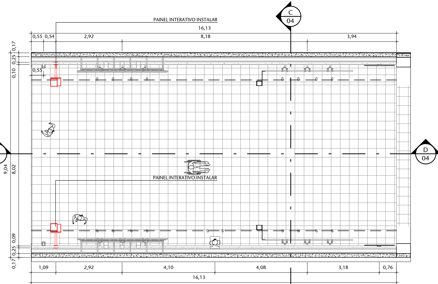
2 SITUAÇÃO PROPOSTA - TRECHO B ESCALA 1 : 100
