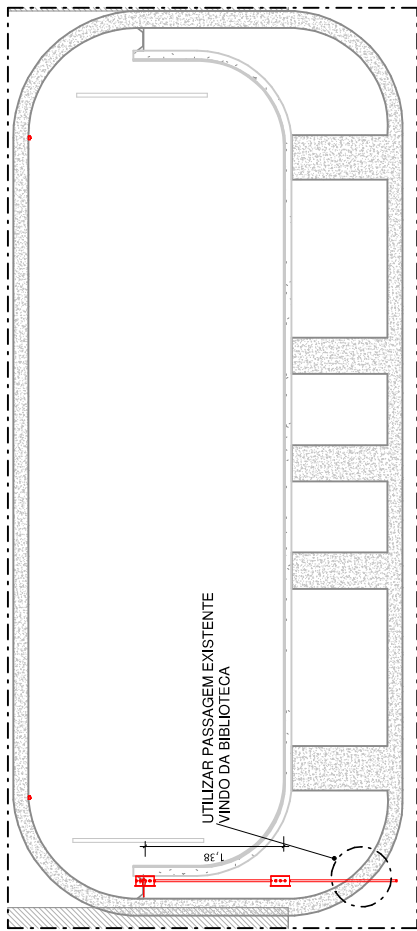
1 Corte 01 ESCALA 1:50
