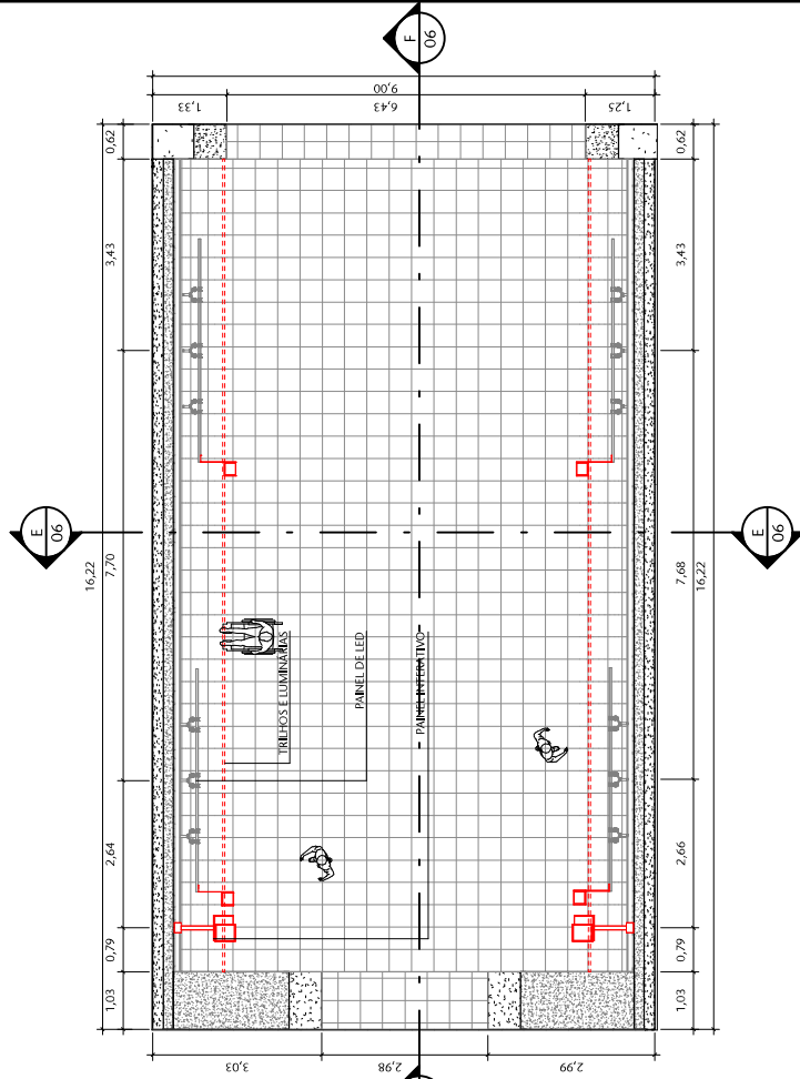
2 SITUÇÃO PROPOSTA- TRECHO C
