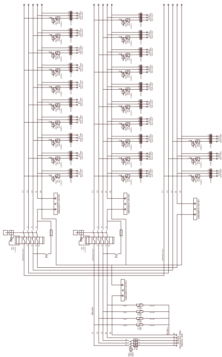
DIAGRAMA UNIFILAR ESCALA 1:8
