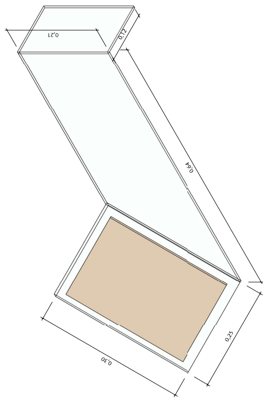
5 DM003 - 3D ESCALA
