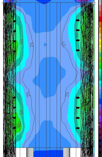
ESTUDO LUMINOTÉCNICO
