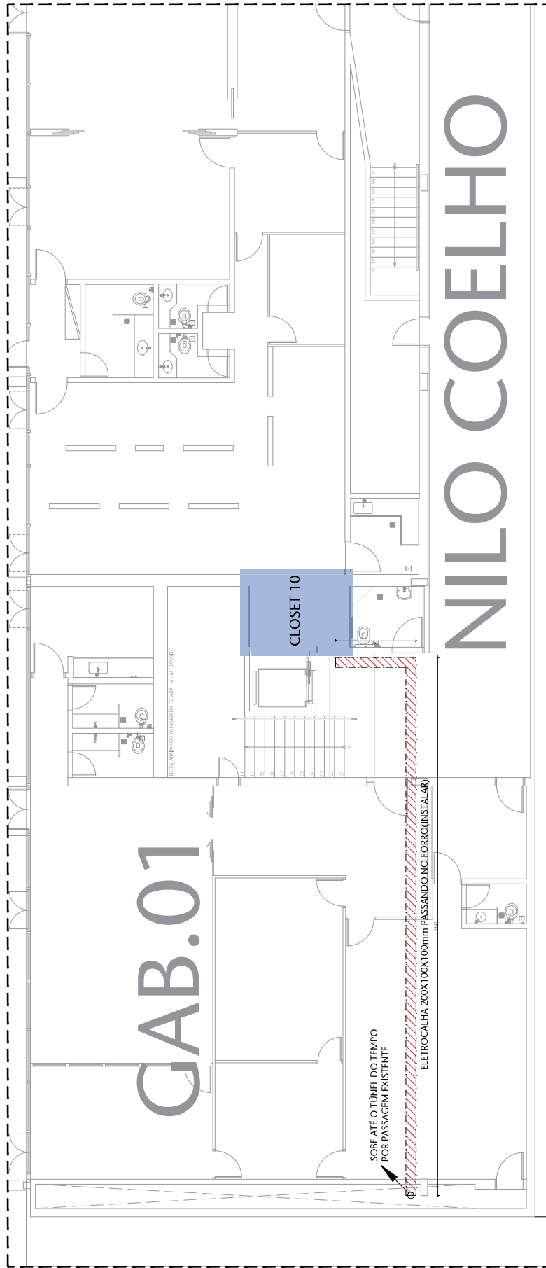
01 PLANTA BAIXA - TÉRREO ALA NILO COELHO ESCALA 1/75
