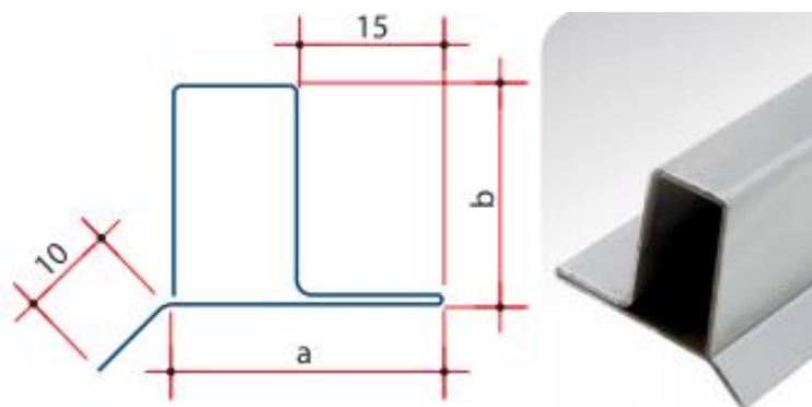
Perfil Cadeirinha Fechada Máximo Ar
