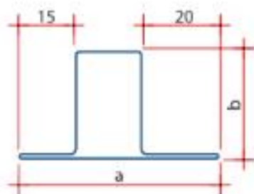
Perfil “T” Dobrado Máximo Ar Abas Desiguais
