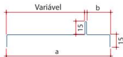
Perfil Marco Vincado
