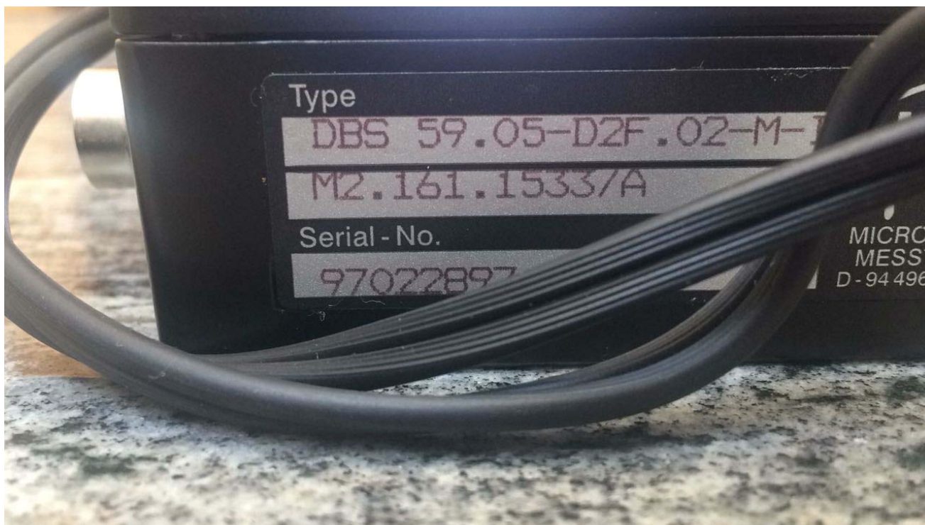
Foto 2 – N° de série e código das peças queimadas.
