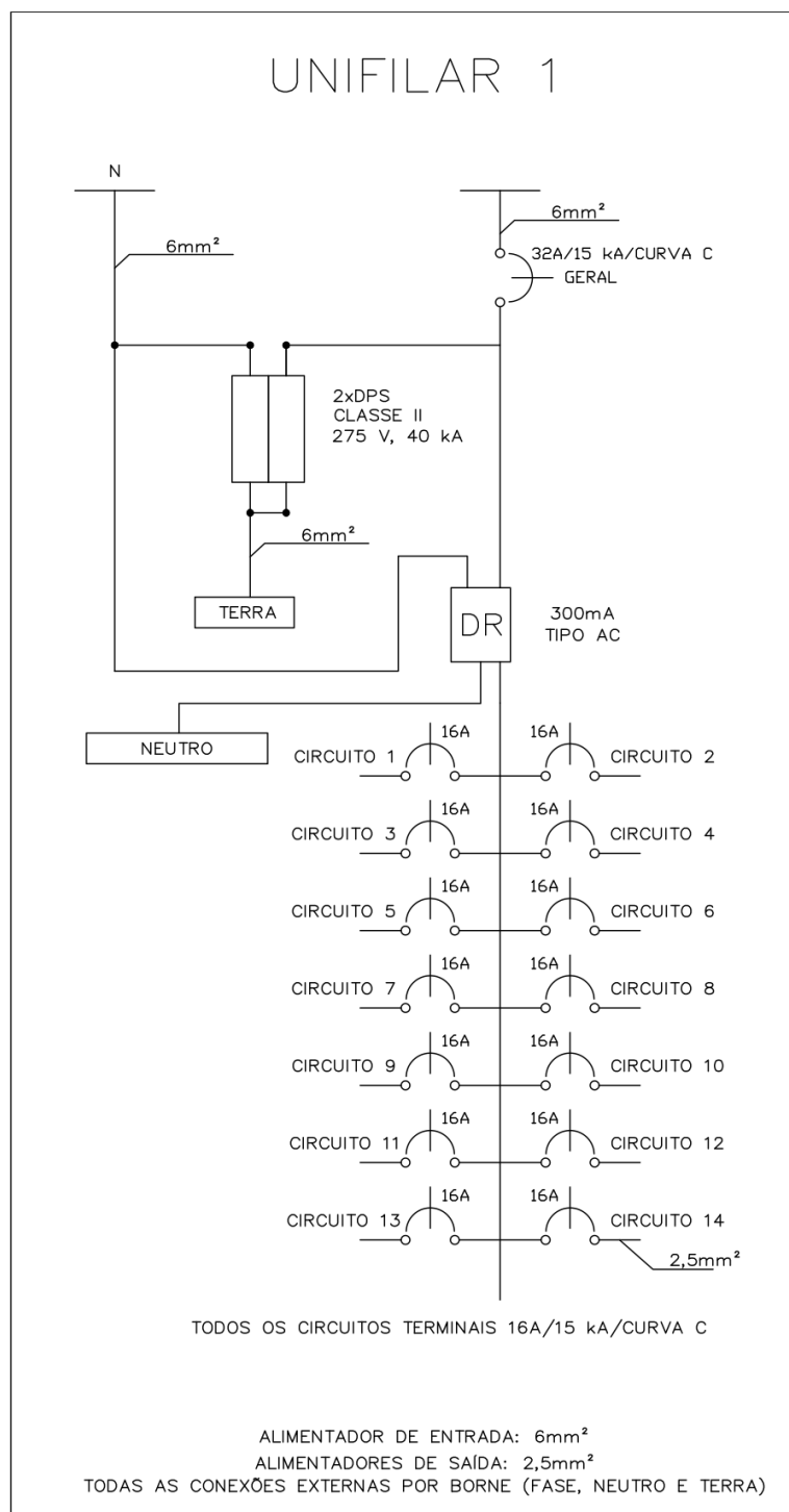
Figura 1 - Diagrama elétrico unifilar do quadro "terminal"
