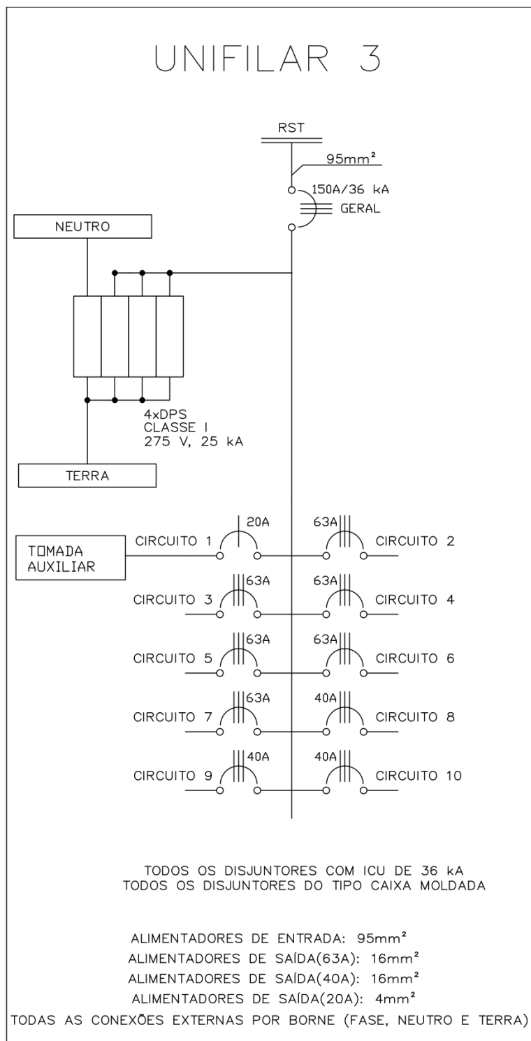
Figura 3 - Diagrama elétrico unifilar do quadro “geral”
