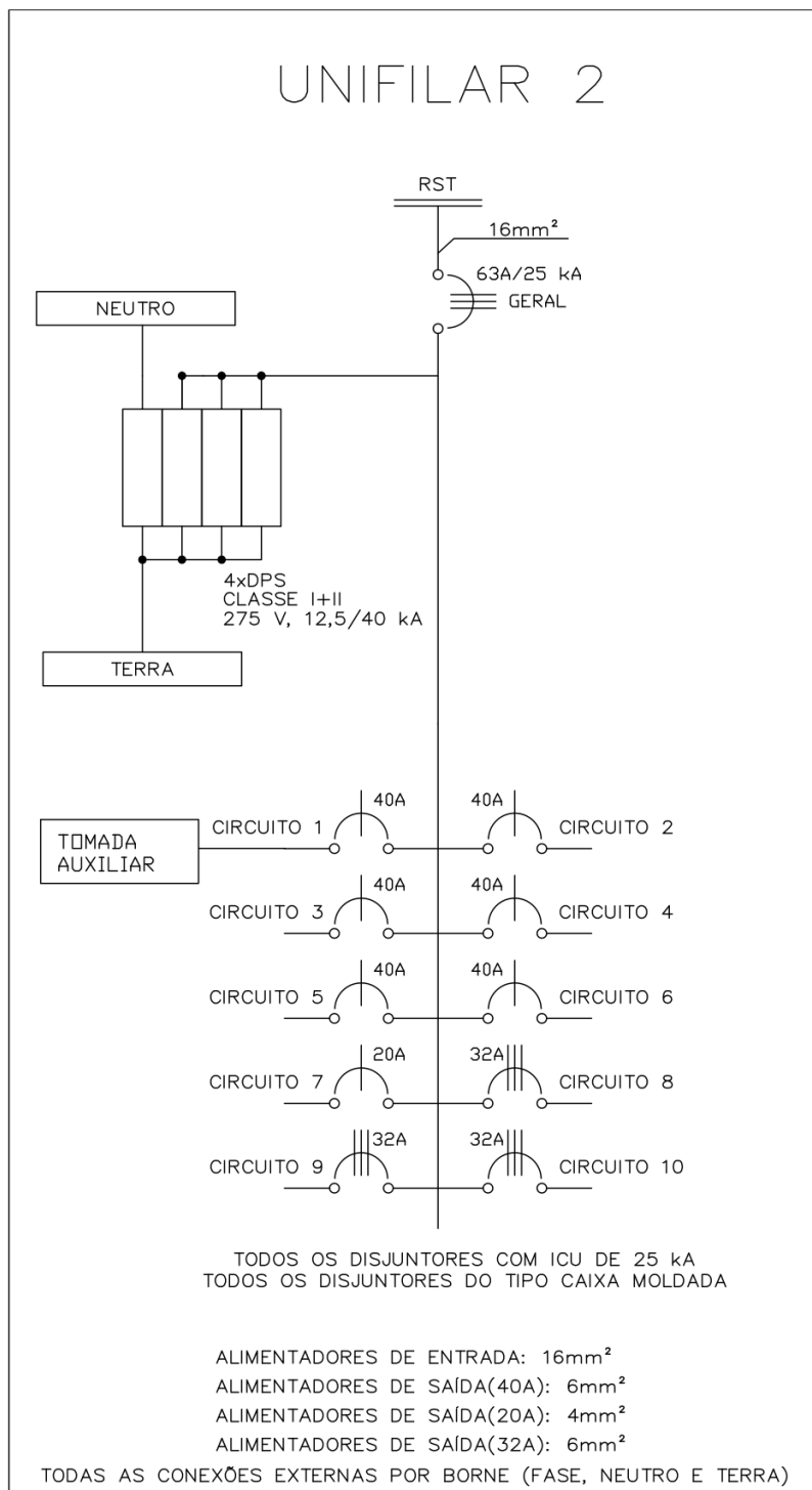
Figura 2 - Diagrama elétrico unifilar do quadro “distribuição”
