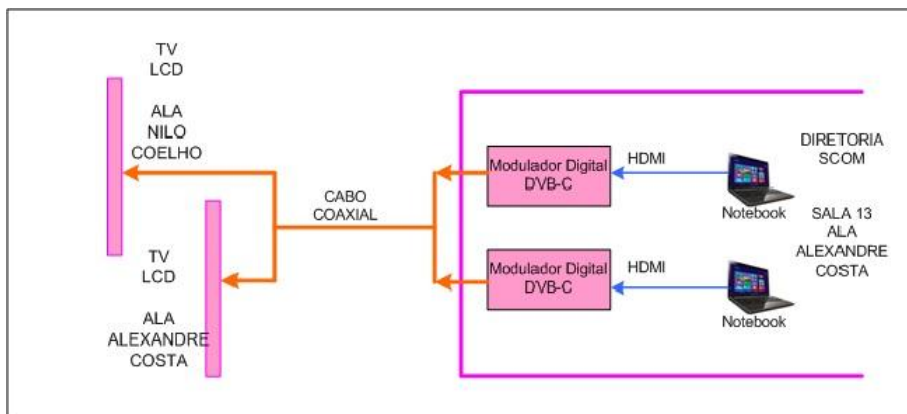
Figura 1 - Conexões de Vídeo entre Televisores
