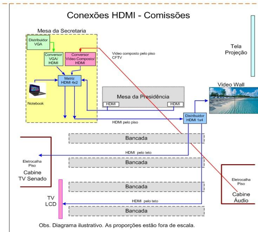
Figura 2 - Conexões HDMI - Comissões
