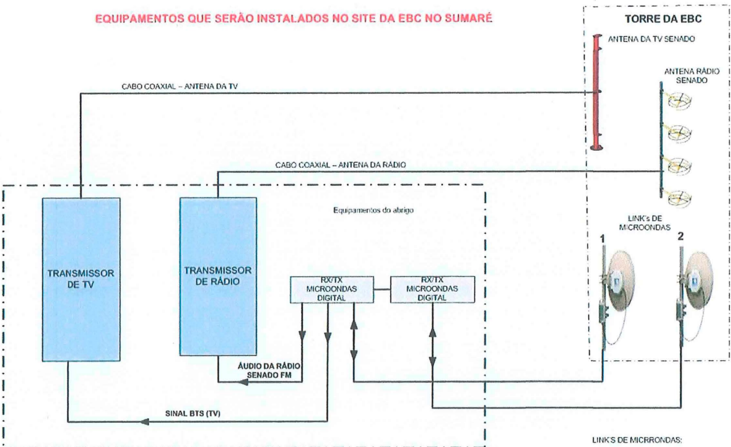
DIAGRAMA EM BLOCOS DA INSTALAÇÃO DA RÁDIO E TV SENADO NO ABRIGO DA EBC
